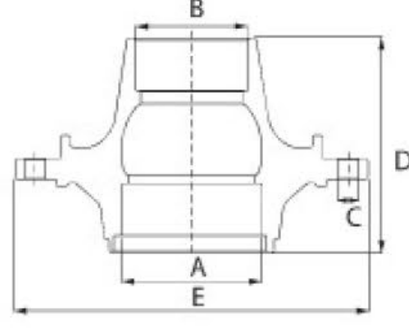
AXOR-ACTROS DİSKLİ ÖN PORYA GÖBEĞİ KİT (2008 SONRASI) WHEEL HUB KIT
