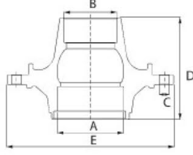
DAF XF-CF DİSKLİ ÖN PORYA KİT (2010 VE SONRASI) WHEEL HUB KIT
