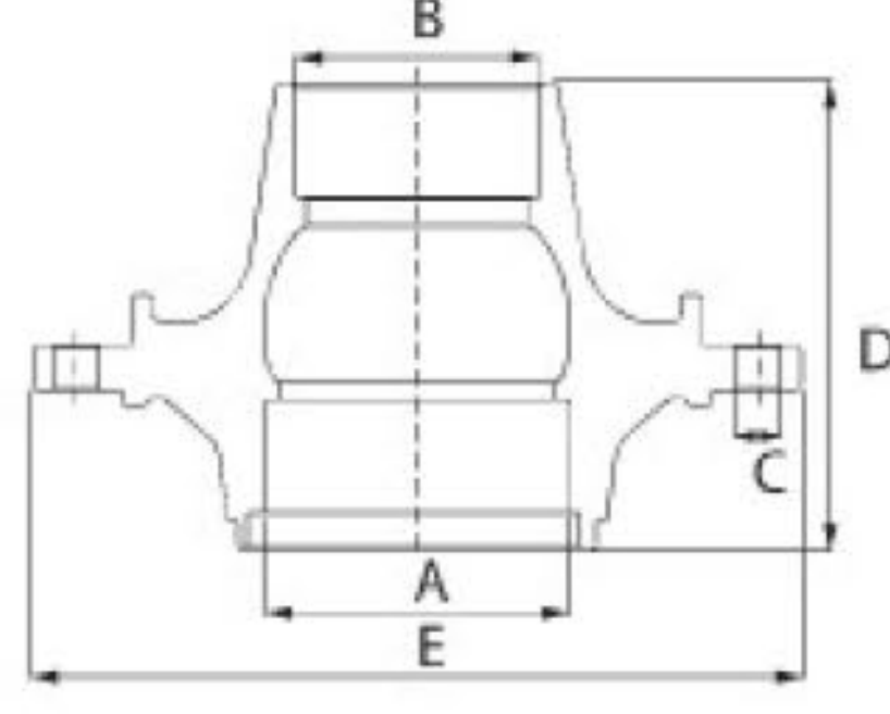
SAF DİNGİL JANT TAŞIYICI FLANŞ FLANGE
