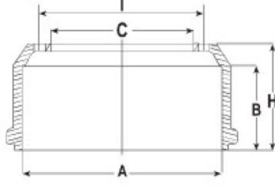
ISUZU - 5 TON ÖN (FRONT)
