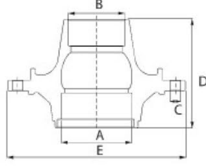
TRAVEGO DİSKLİ ÖN PORYA GÖBEĞİ (2008 SONRASI) HUB UNIT (FOR BRAKE DISC)
